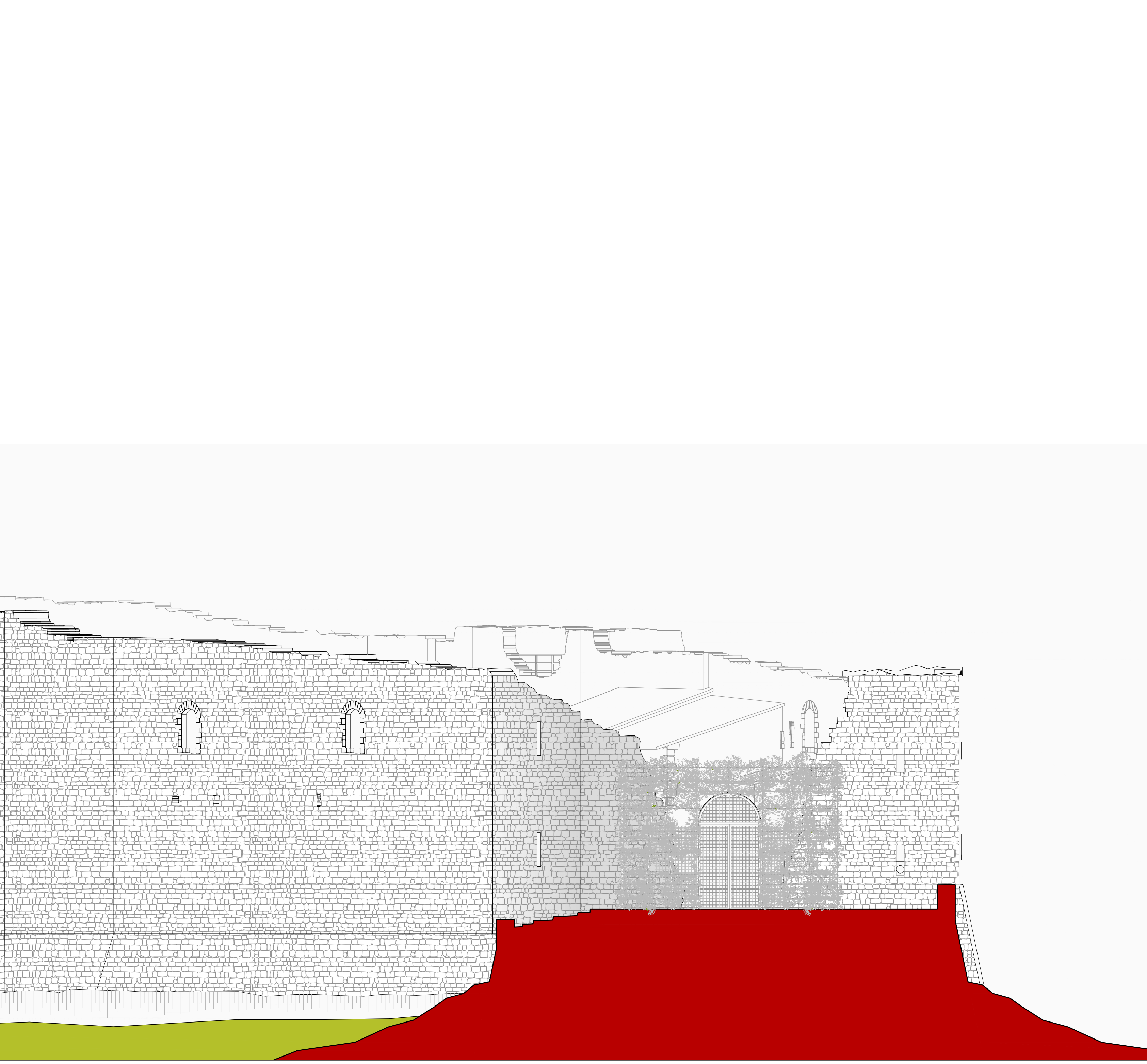
PROSPETTO ESTERNO LATO OVEST
