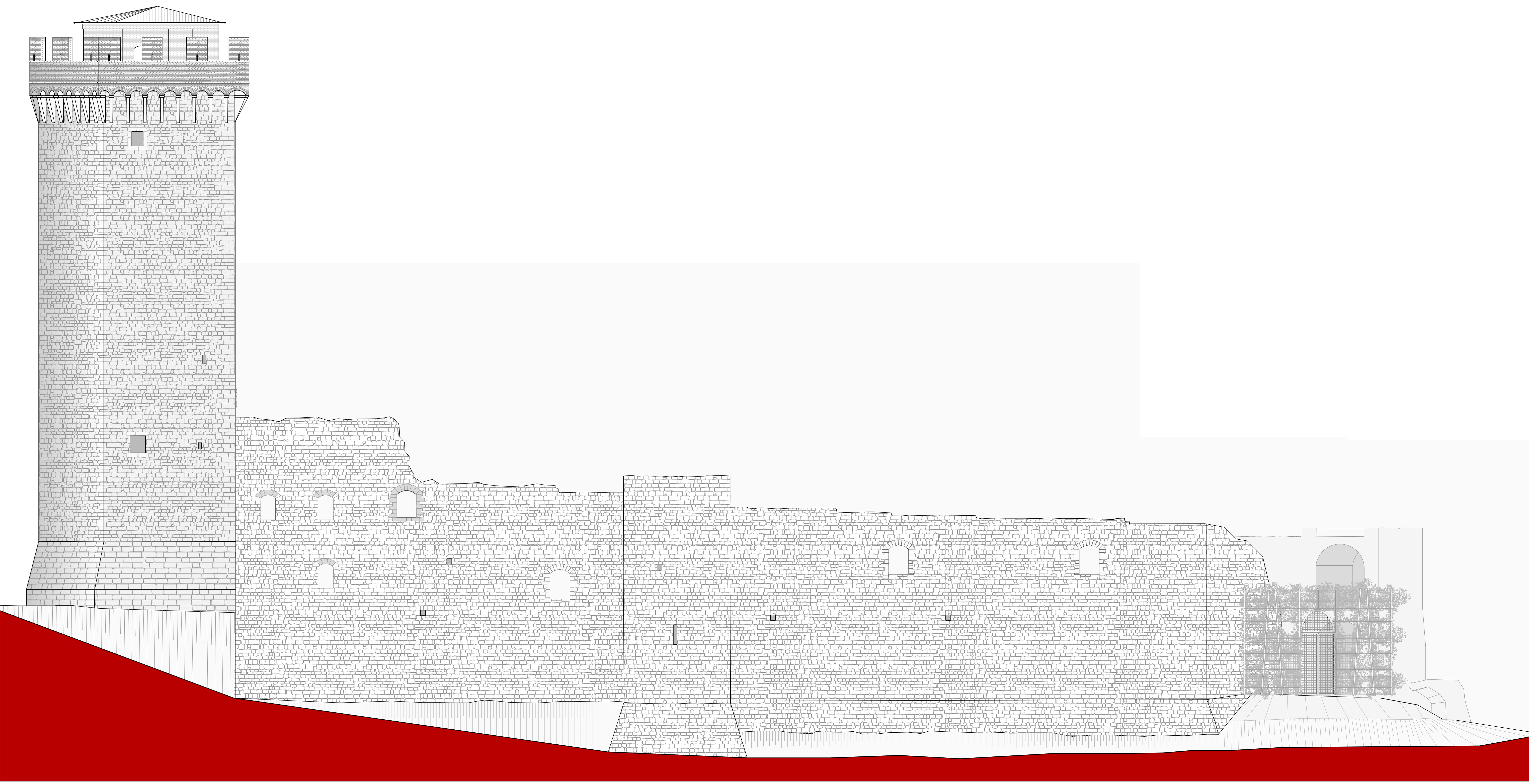
PROSPETTO ESTERNO LATO NORD
